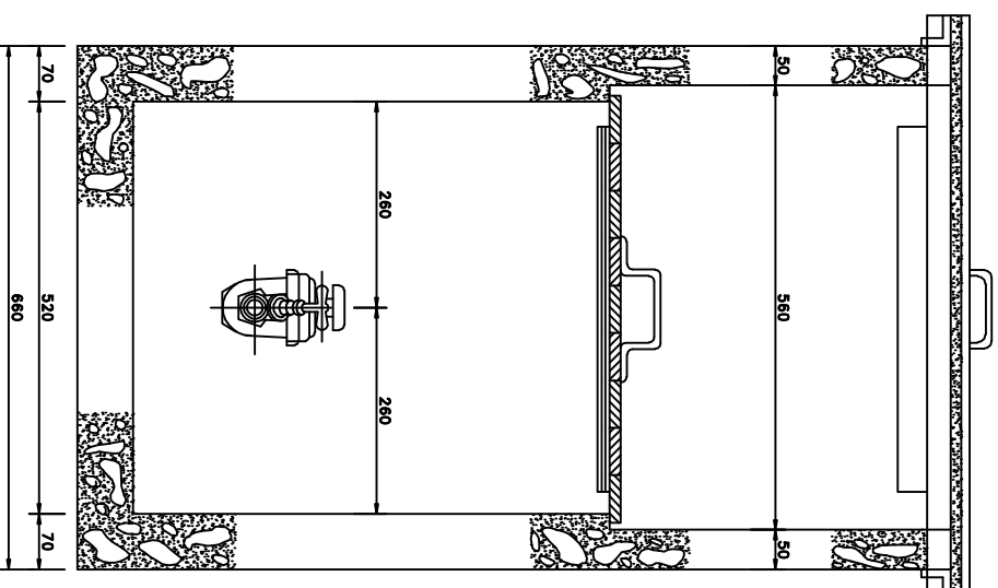
ZIJAANZICHT
