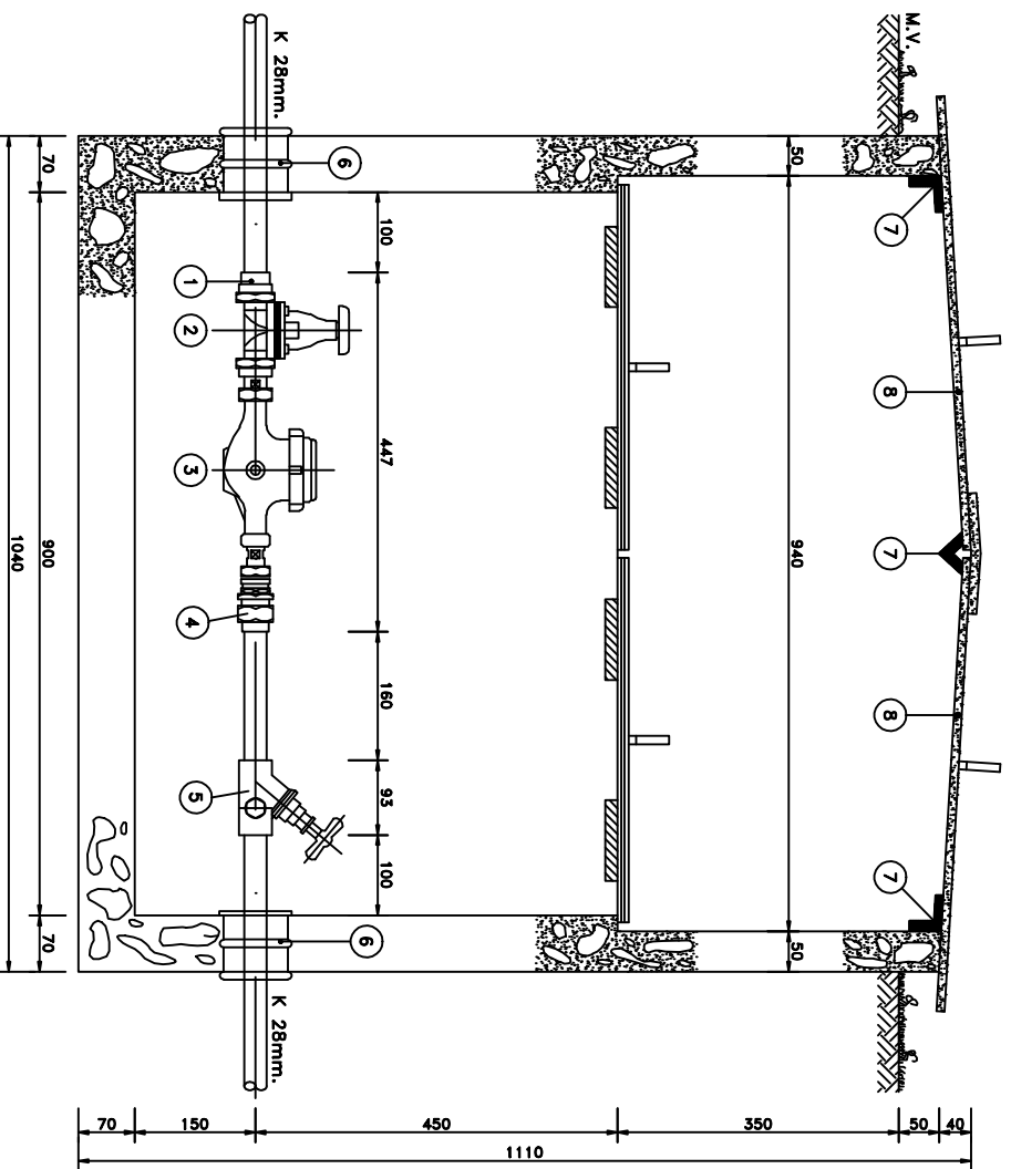
VOORAANZICHT
