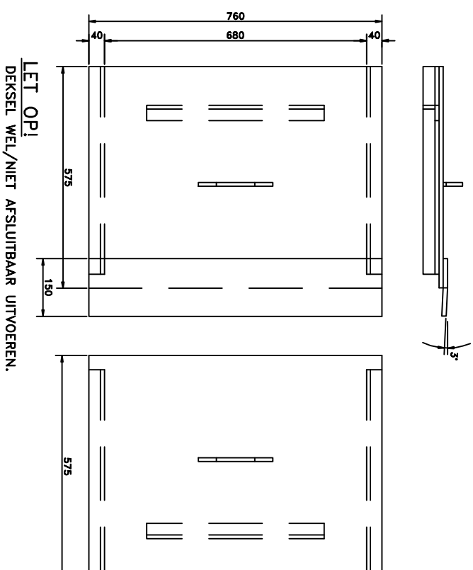
BOVENAANZICHT PUTDEKSELS
